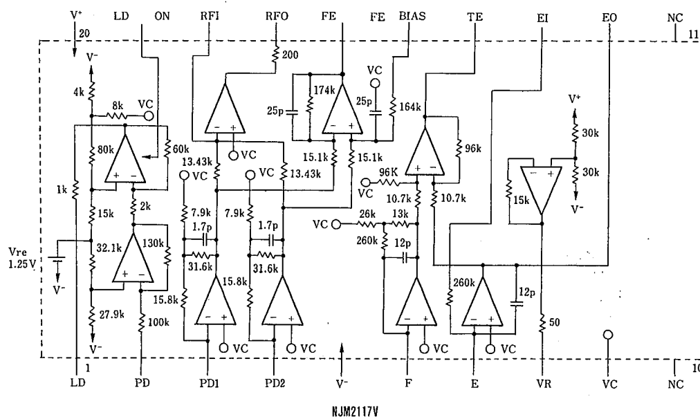
NJM2117V
