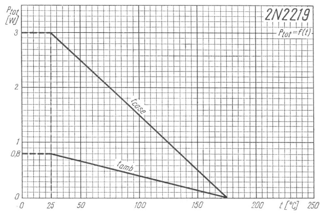
Rys. 1-1167. Zależność całkowitej mocy strat od temperatury
