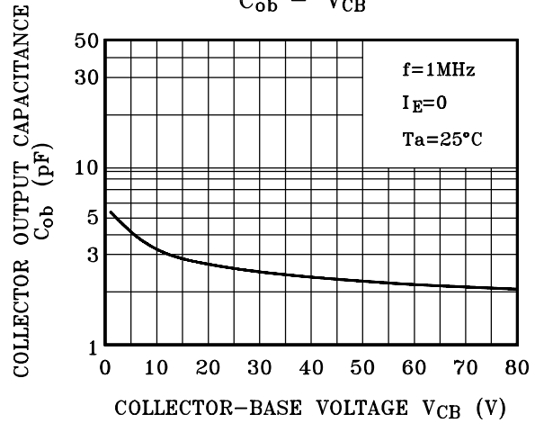
C_{ob} - V_{CB}
