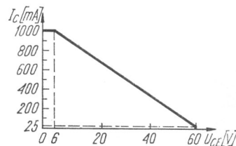
Rys. 1-890. Dopuszczalny zakres pracy
