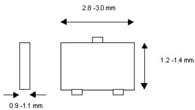
SOT- 23
