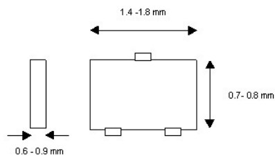
SOT- 416/SC- 90
