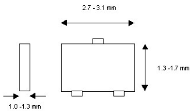
SC- 59
