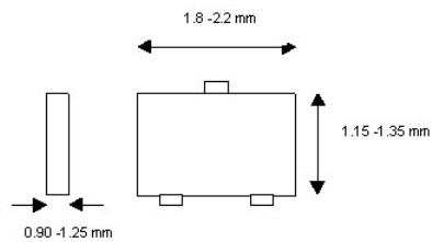
SOT- 323/SC-70
