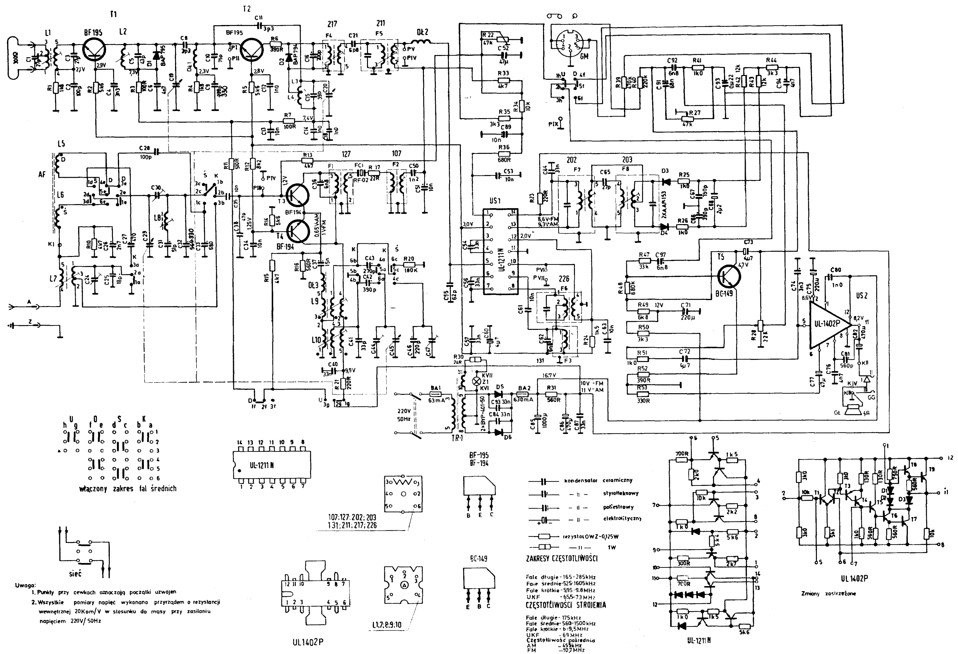
Rys. 3: Schemat ideowy odbiornika radiowego „ALBA DMP-408”
