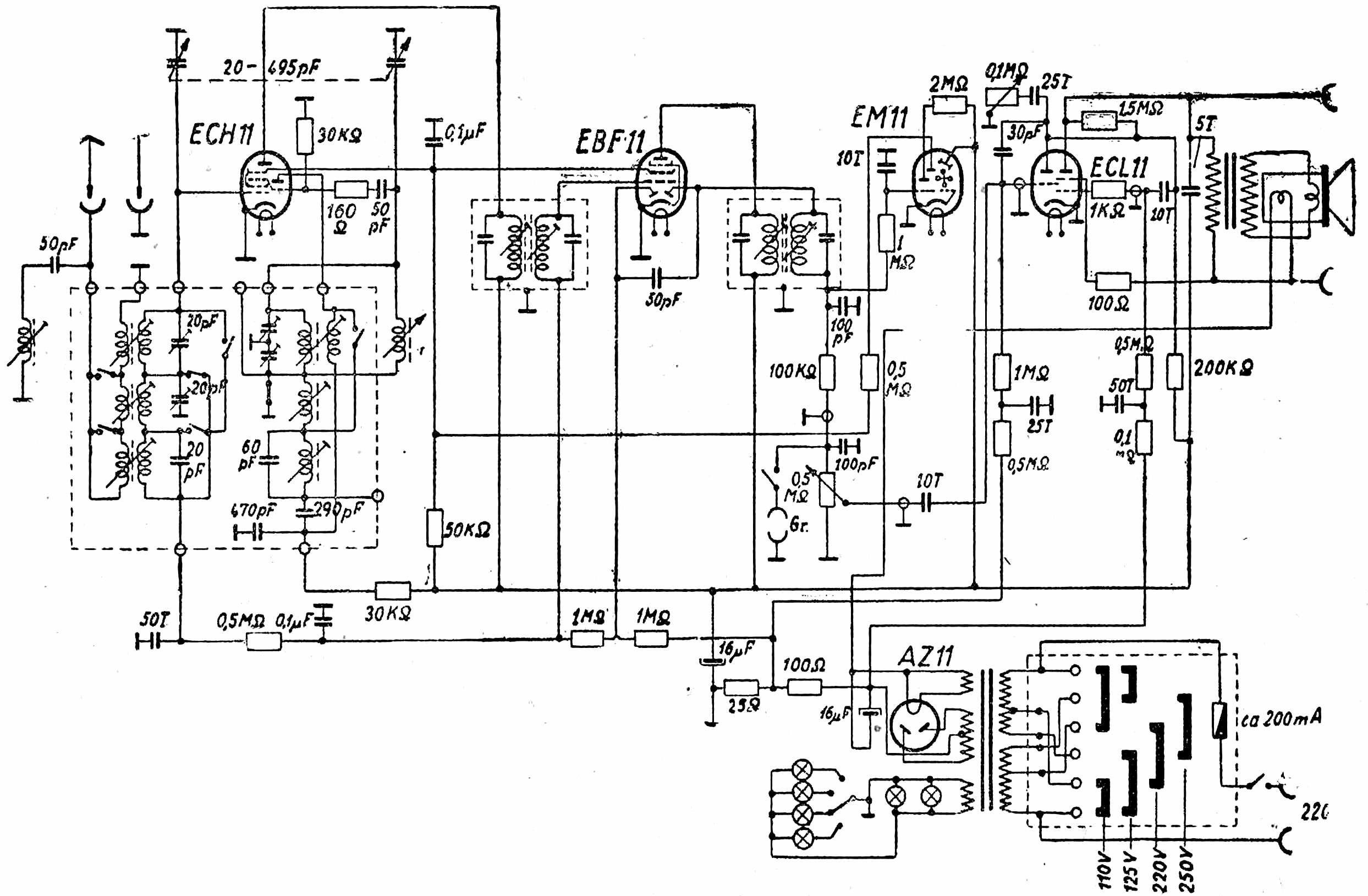
Schemat odbiornika EAK
