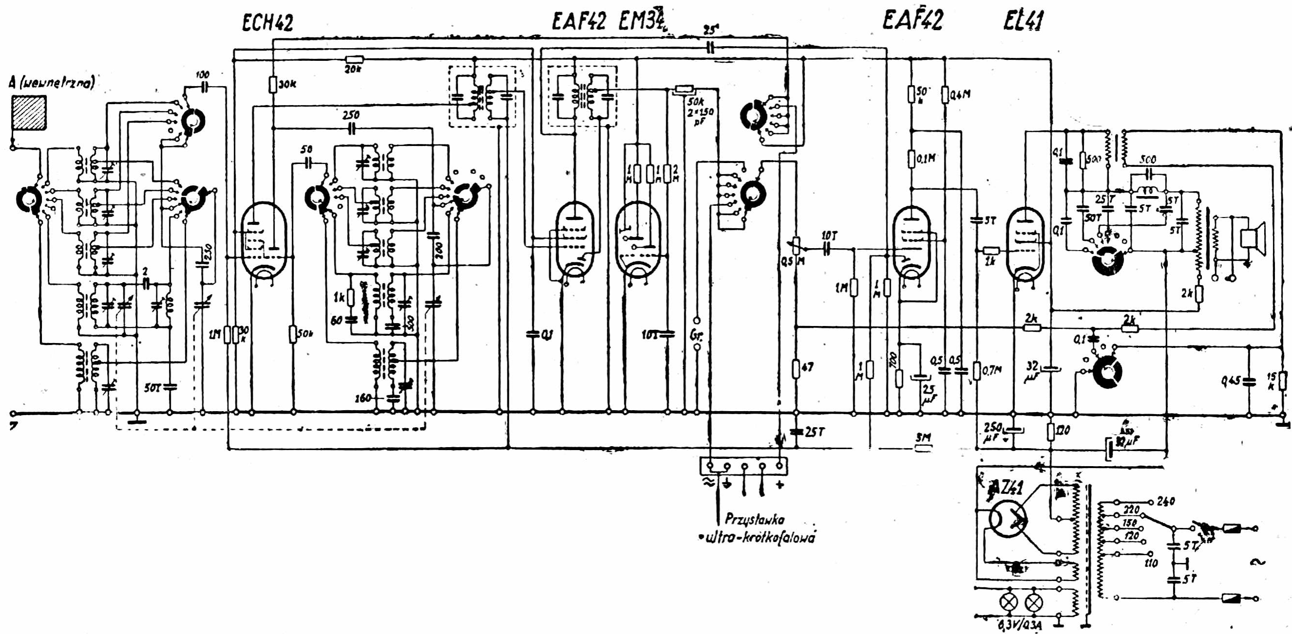
Schemat odbiornika „Ferrando“
