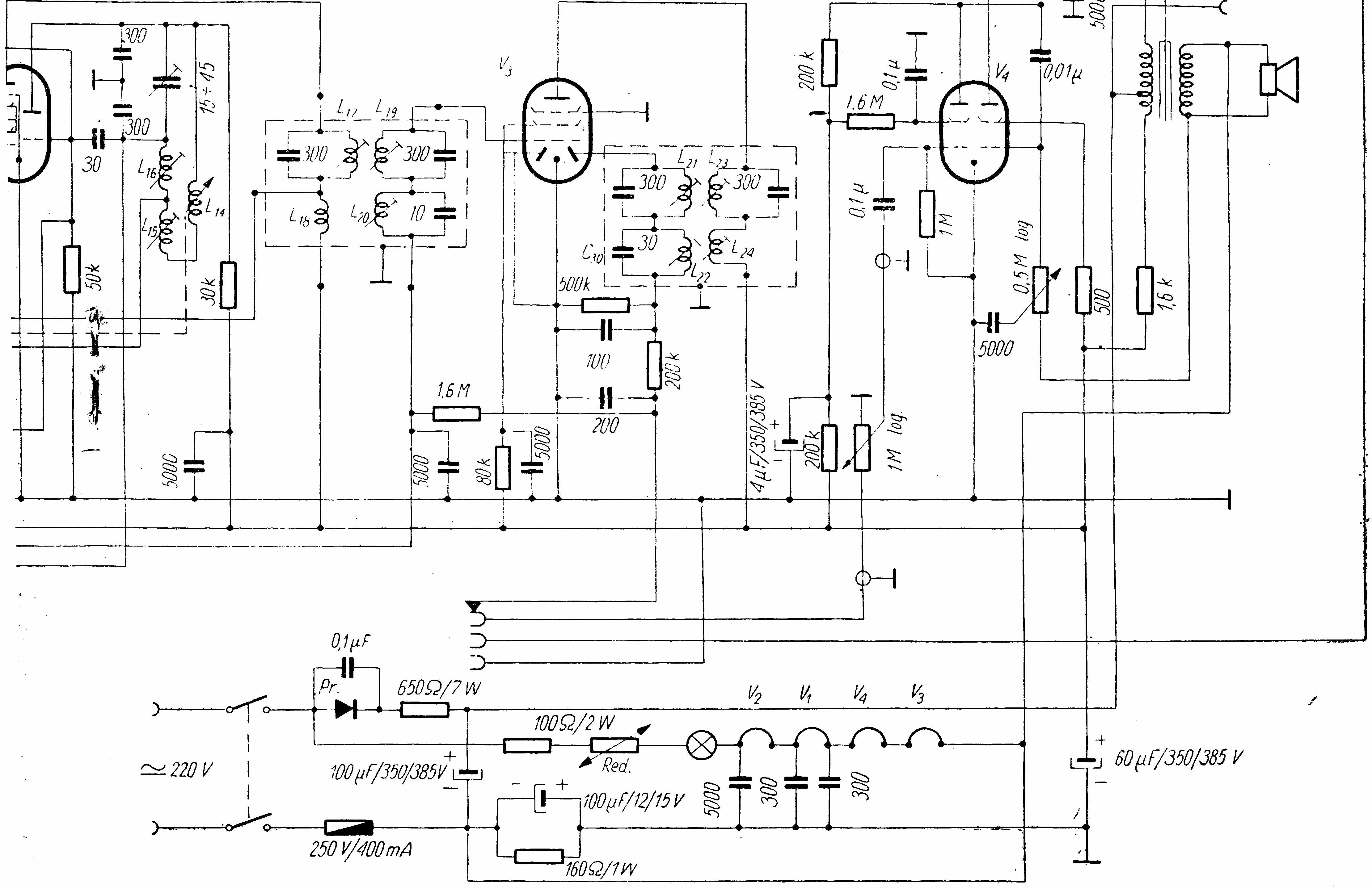
Schemat ideowy odbiornika Ilmenau 675/55 GWU
