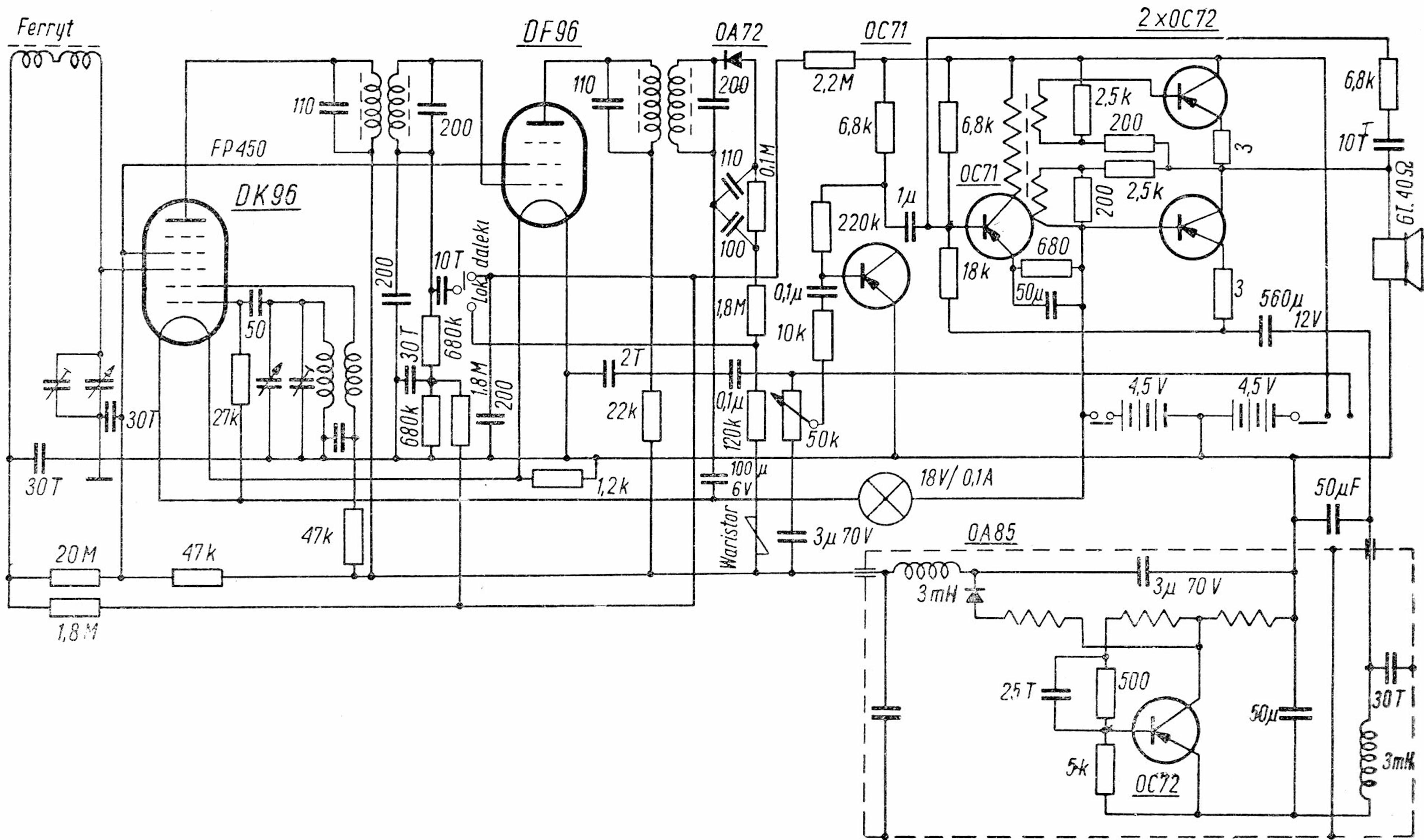
Schemat ideowy odbiornika „Ingelen TR56“
