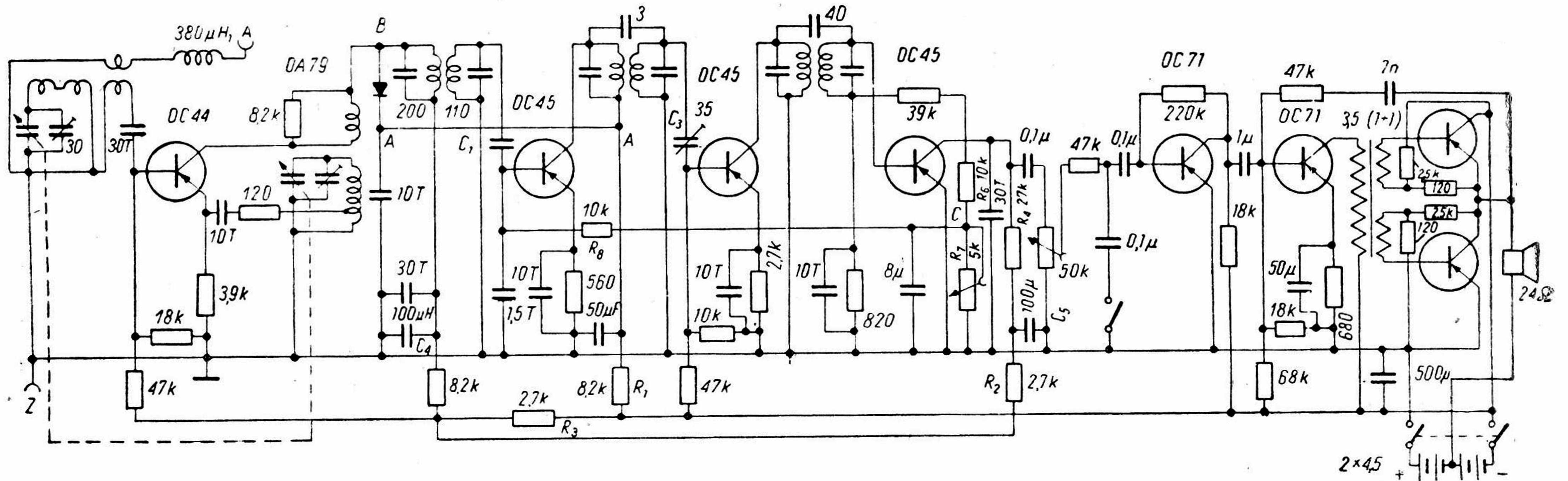
Schemat ideowy odbiornika Ingelen TRV-100
