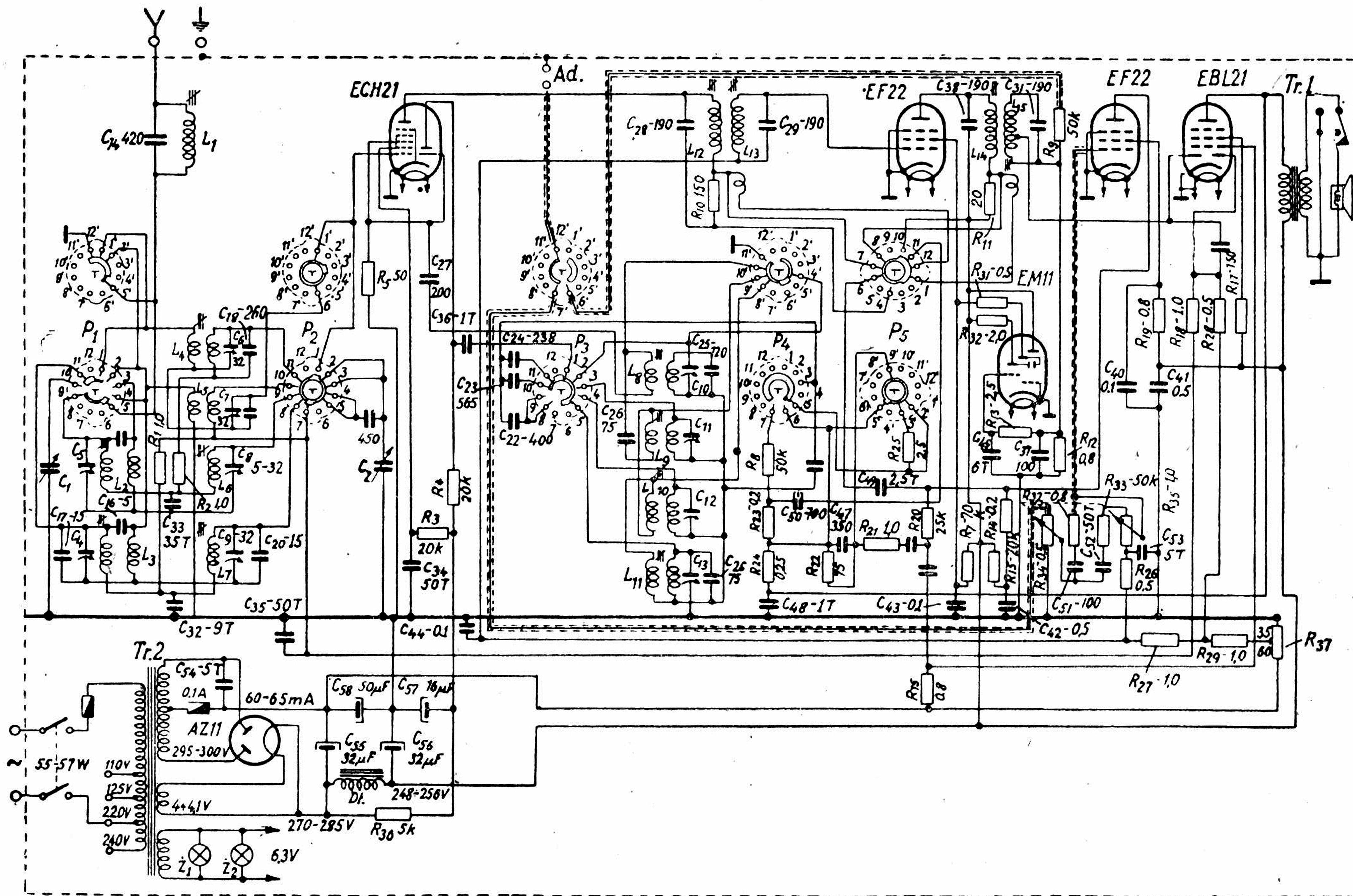
Schemat ideowy odbiornika „Kongress“
