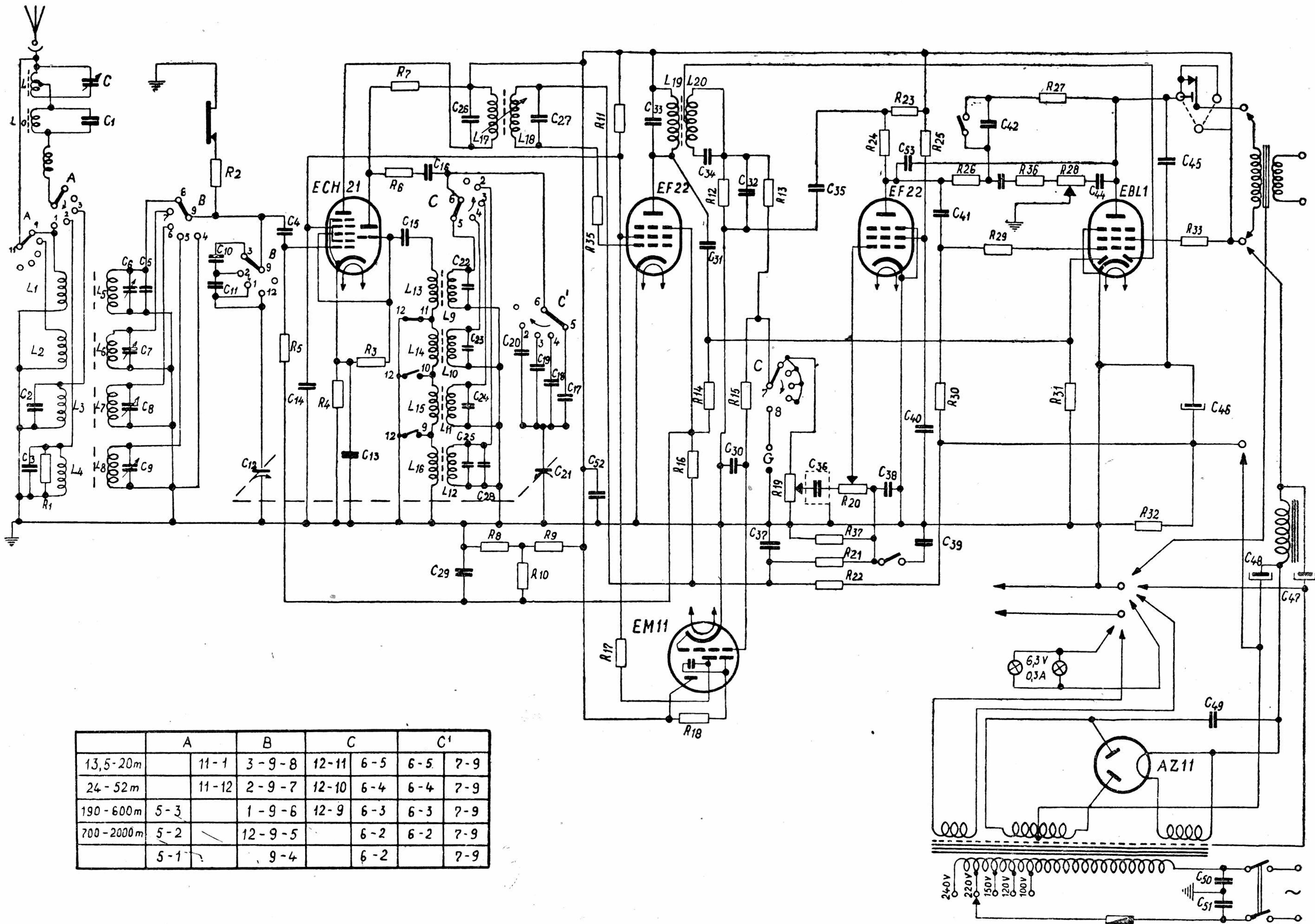
Schemat ideowy odbiornika „Liberator“
