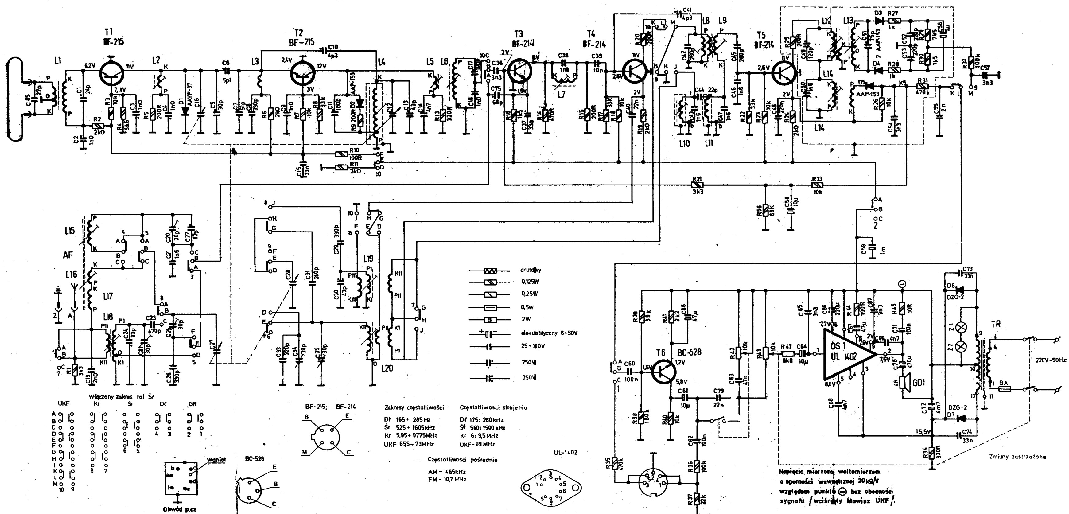
SCHEMAT IDEOWY OR „LUDWIK” NA OBWODZIE SCALONYM
