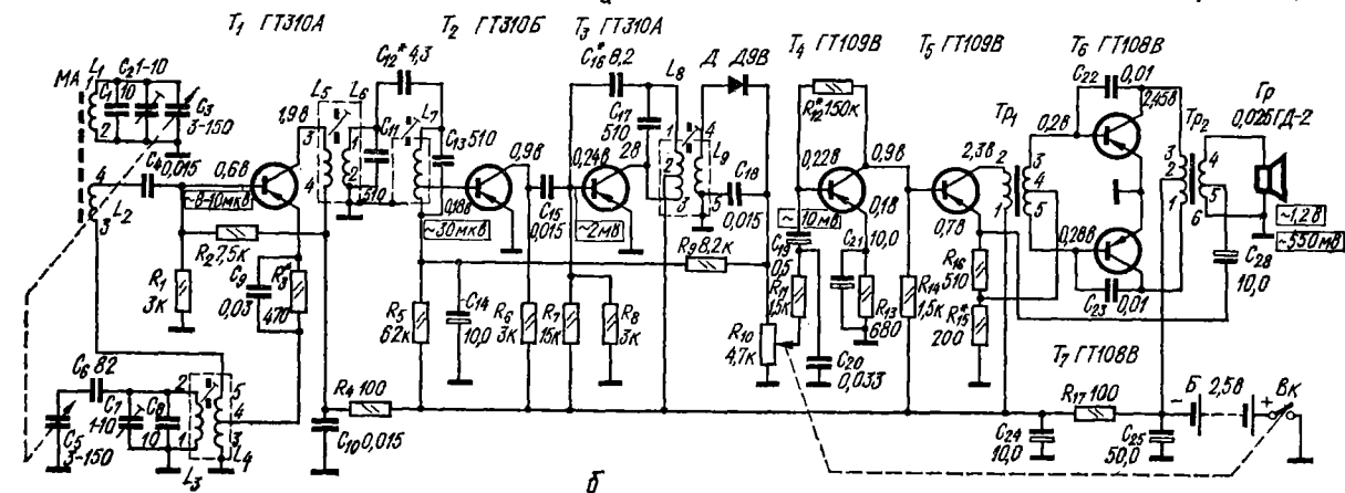
Принципиальная электрическая схема радиоприемников «Рубин» (а) и «Рубин-2» (б) (с диапазоном ДВ)
