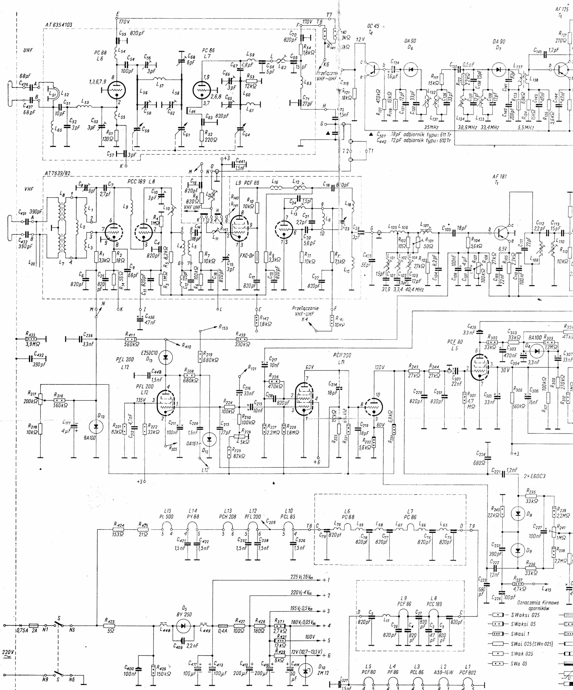
Rys. XVII.95. Schemat elektryczny odbiornika lampowo-tranzystorowego
